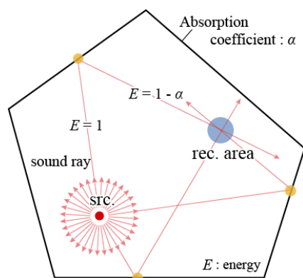
図2. 音線法
